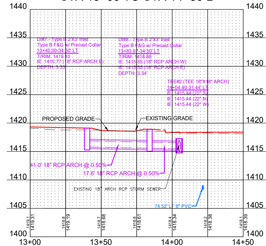
STA 13+00 TO STA 14+50 L
