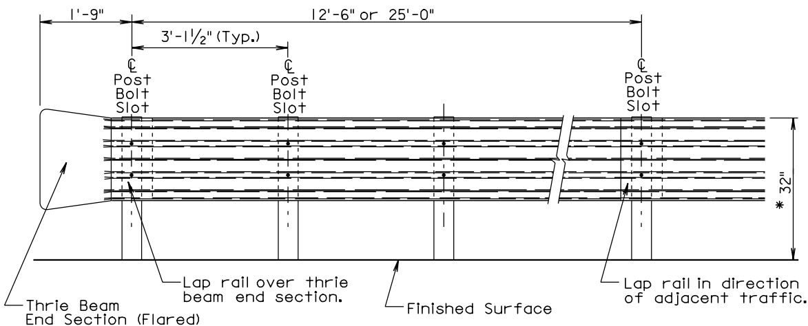
ELEVATION
