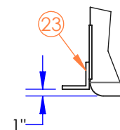
ANCHOR LUG DETAIL (NOT TO SCALE)
