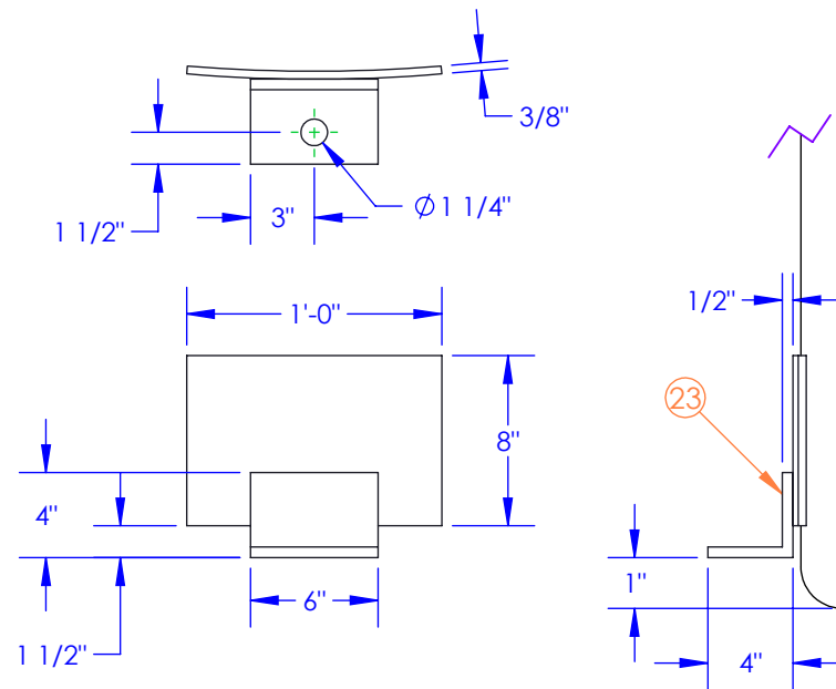
ANGLE ANCHOR LUG DETAIL (NOT TO SCALE)
