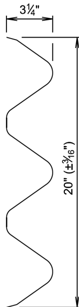
VIEW A-A
